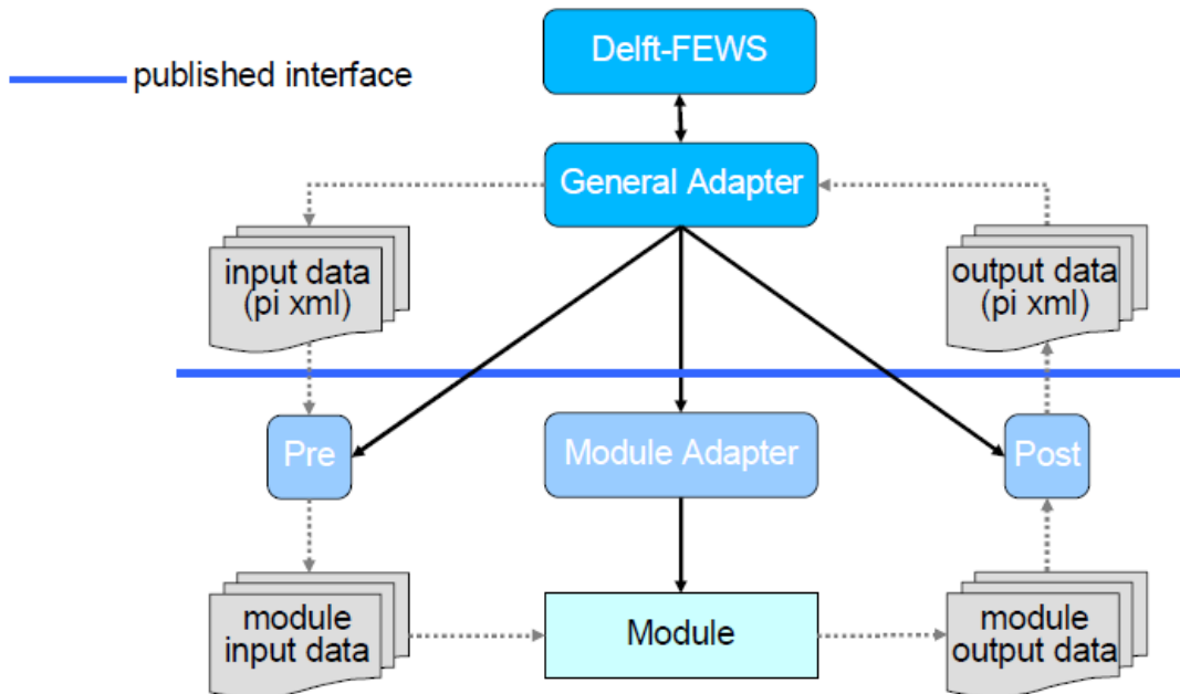
Figuur 2.12 Overzicht integratie van externe modellen in het Nationaal Water Model
