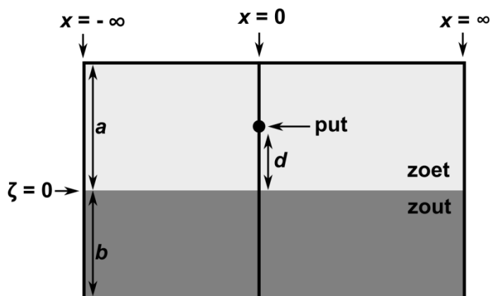
Figuur 3.22: Modelopzet in dwarsdoorsnede voor vergelijking (6).
