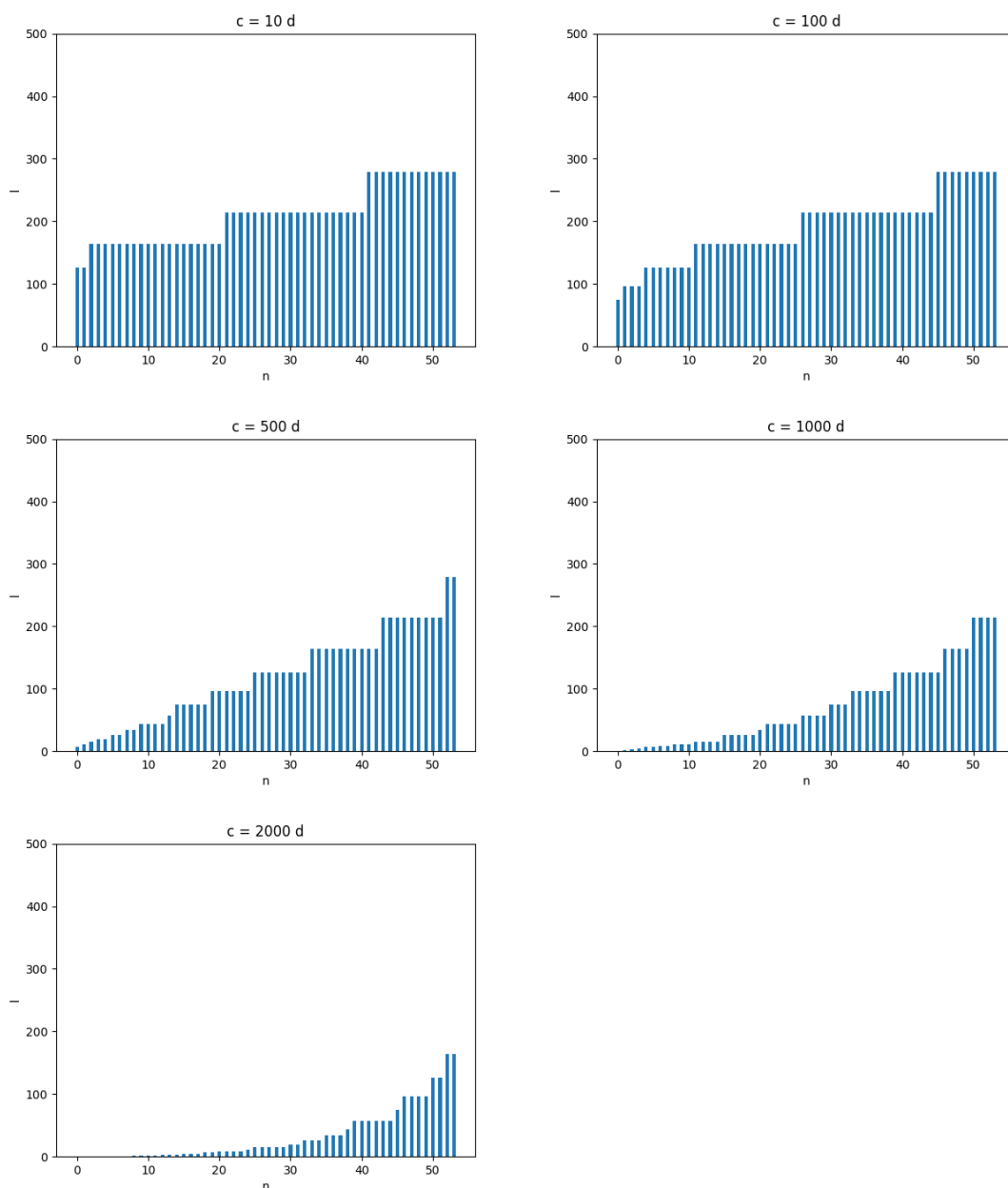
Figuur 4.57: Verlagingsbereik van 5 cm ( l ) bij toepassing van alle parametercombinaties, gesorteerd op waarden van l .
