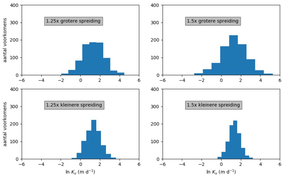
Figuur 4.19: Verdeling van K_v in de random gegenereerde set met verschillende waarden voor de standaarddeviatie ten opzichte van de standaard deviatie uit de GeoTOP Zeeland series.
