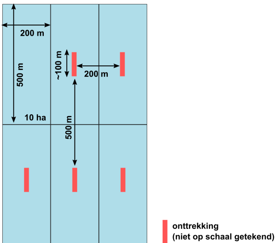
Figuur 2.4: Vastgesteld buffergebied rondom een landbouwonttrekking (blauwe vlakken). In deze situatie bevindt de dichtstbijzijnde onttrekking zich op 200 m van een andere onttrekking. In de richting loodrecht op deze onttrekking moet zich een onttrekking op (minimaal) 500 m afstand bevinden om tot 10 ha (totale oppervlakte buffergebied) te komen. De lengte van de onttrekking is in dit geval ~80-100 m, gebaseerd op praktijksituaties. In de regelgeving is echter geen expliciete eis ten aanzien van de lengte van de onttrekking meegenomen.
