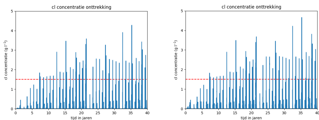
Figuur 4.71: Verloop van de chlorideconcentratie in de onttrekking van het scenario zonder freatische grondwateraanvulling met de open rand dichtbij (links, op 300 m) en veraf (rechts, op 1000 m).
