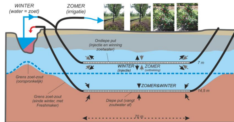
Fig. 10: De Freshmaker injecteert zoet oppervlaktewater in de winter met een ondiepe HDDW en vangt zout water af met een diepere HDDW. In droge periodes kan de ondiepe HDDW zoet water leveren aan bassin of druppelirrigatie.
