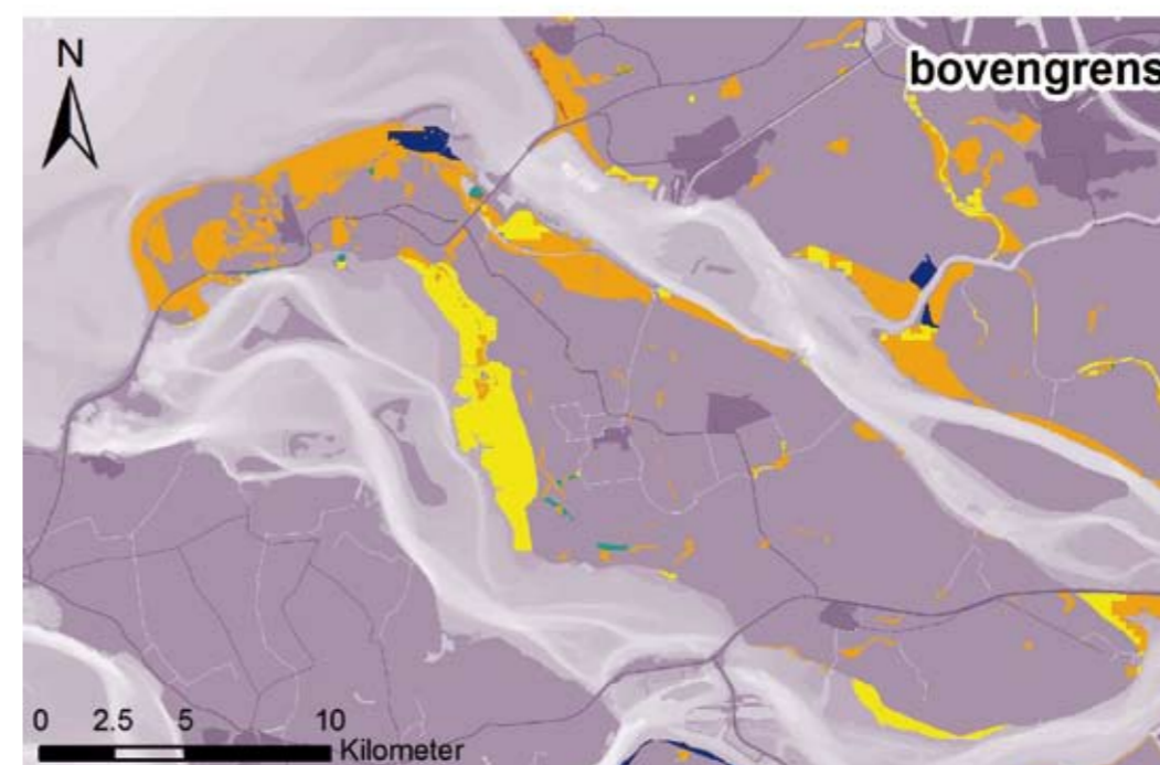
Figuur 16 De optimale concentratie chloride (boven) en de concentratie horende bij de bovengrens (onder: het abiotisch maximum, +2 SD) voor natuurdoeltypen op Goeree-Overflakkee.
