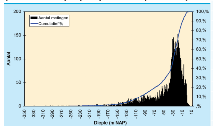
Afb. 2: Aantal metingen en percentage van het totaal als functie van de diepte.
