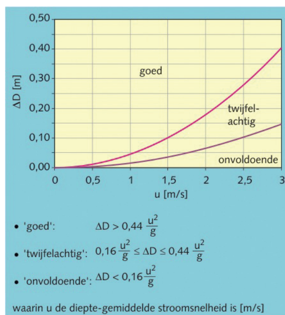
Figuur 8 - 2.9 Eenvoudige toetsing toplaaginstabiliteit op langsstroming
