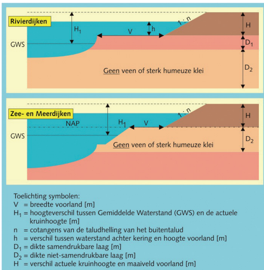
Figuur 5 - 4.17 Geometrische toets Macrostabiliteit buitenwaarts
