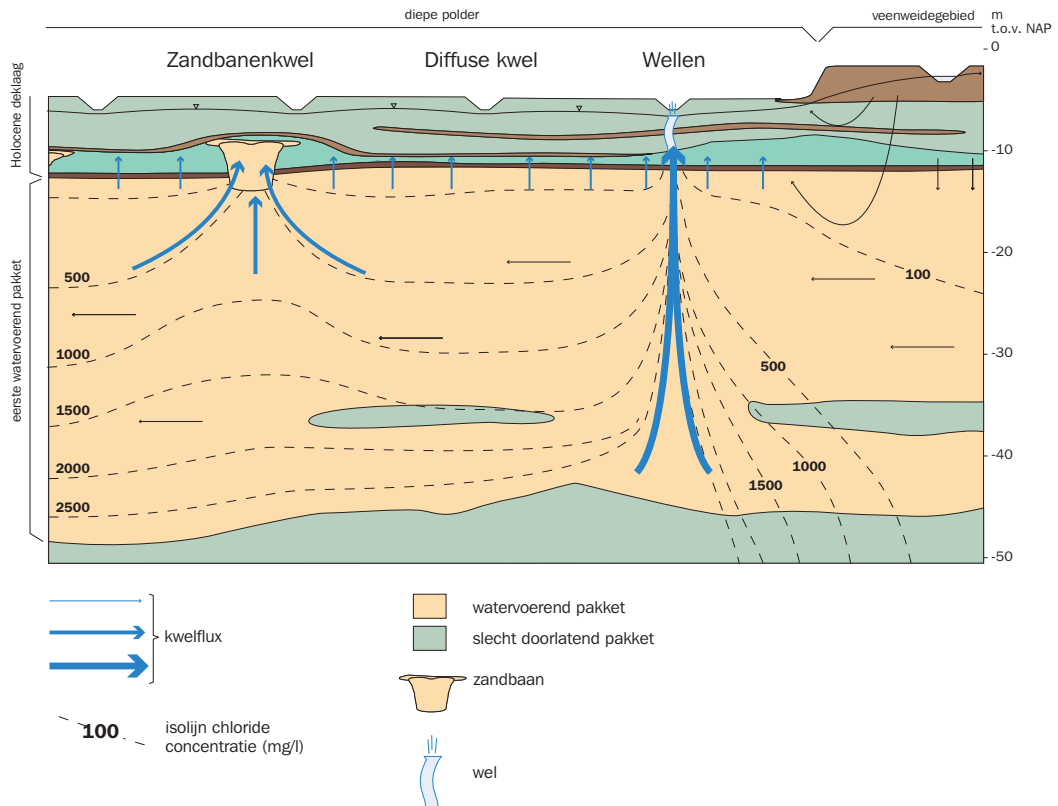
Fig. 1. Drie typen kwel in een diepe polder met verschillende fluxen en zoutgehaltes
